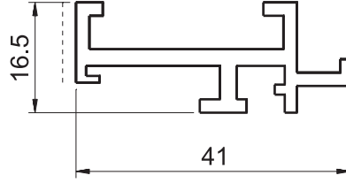
2402 0.531 kg/m
