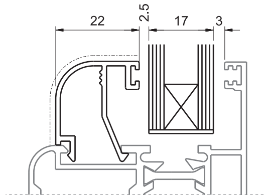
2071 0.299 Kg/m
