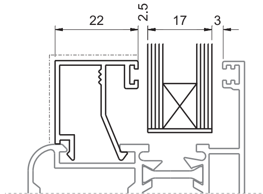
2072 0.313 Kg/m
