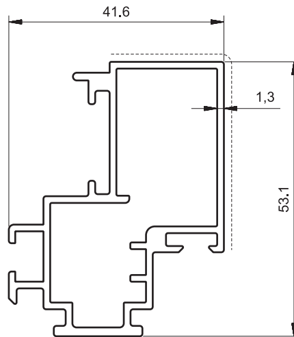
3461 0.907 Kg/m
