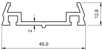
4015 0.493 Kg/m
