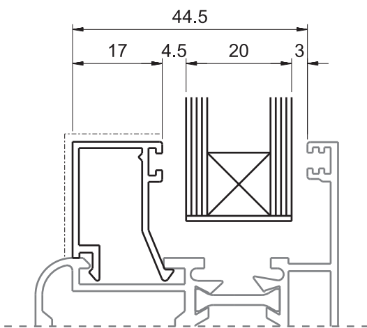
1965 0.269 Kg/m
