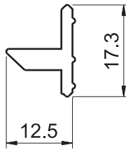
2405 0.205 kg/m
