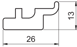
2401 0.449 kg/m
