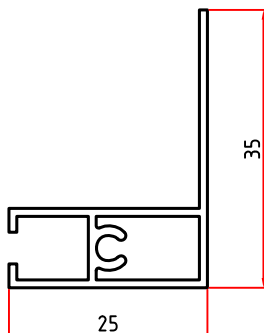
6090 0,298 Kg/m
