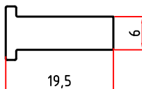
5323 0,352 Kg/m
