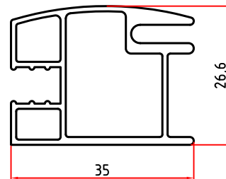
3085 0,594 Kg/m
