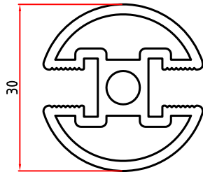
5321 0,784 Kg/m
