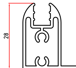
3093 0,452 Kg/m
