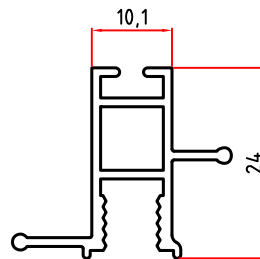
2704 0,300 Kg/m
