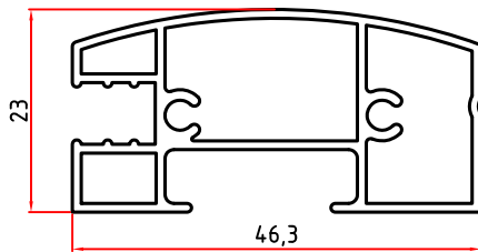
3087 0,596 Kg/m
