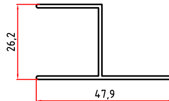
2710 0,406 Kg/m
