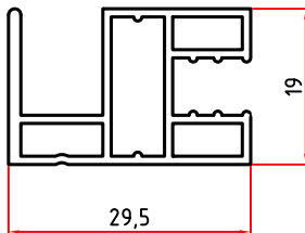
3084 0,422 Kg/m
