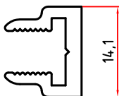
5992 0,206 Kg/m
