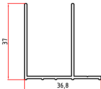
5888 0,372 Kg/m
