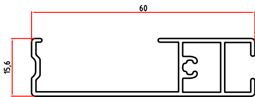
7258 0,470 Kg/m
