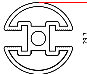
6014 0,751 Kg/m
