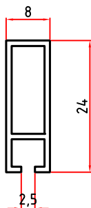
5079 0,181 Kg/m
