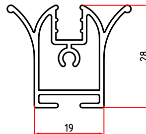
3089 0,525 Kg/m
