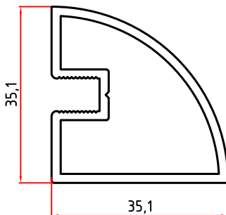
5833 0,697 Kg/m
