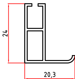
5085 0,220 Kg/m
