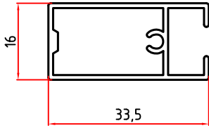
5063 0,325 Kg/m
