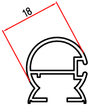
5065 0,234 Kg/m
