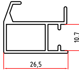
2702 0,311 Kg/m
