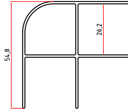
5034 0,709 Kg/m
