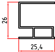
5035 0,298 Kg/m
