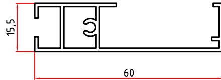
5066 0,464 Kg/m
