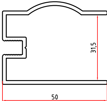
5319 0,772 Kg/m
