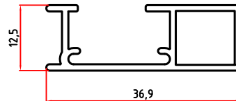
7259 0,315 Kg/m
