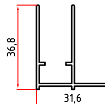
5062 0,372 Kg/m
