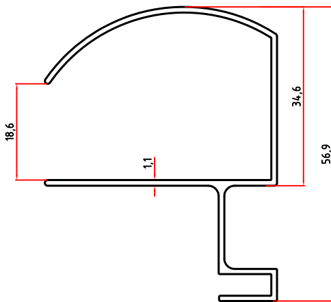
7192 0,518 Kg/m
