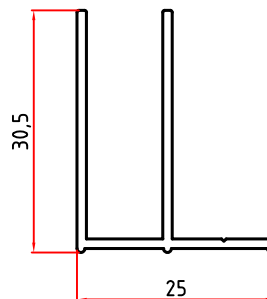
5887 0,285 Kg/m
