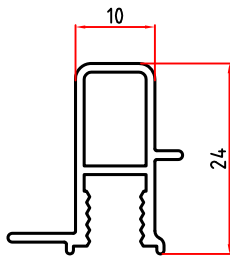
2701 0,255 Kg/m
