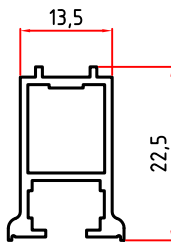
5067 0,289 Kg/m
