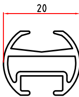
4307 0,277 Kg/m
