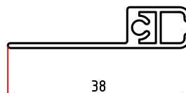
5082 0,219 Kg/m
