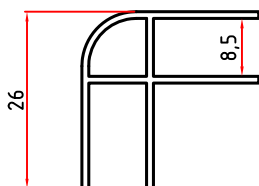
5077 0,275 Kg/m
