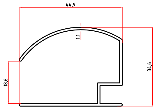
7191 0,413 Kg/m
