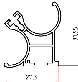
5068 0,392 Kg/m
