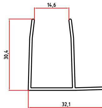
7193 0,283 Kg/m
