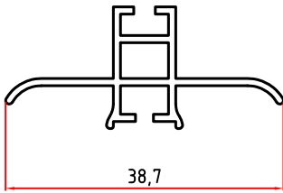
5107 0,251 Kg/m
