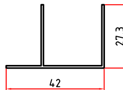
5036 0,269 Kg/m
