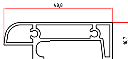
6163 0,527 Kg/m
