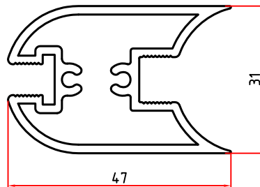
5322 1,005 Kg/m
