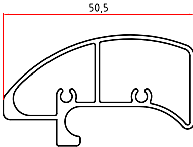
5355 0,653 Kg/m
