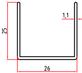
2709 0,239 Kg/m
