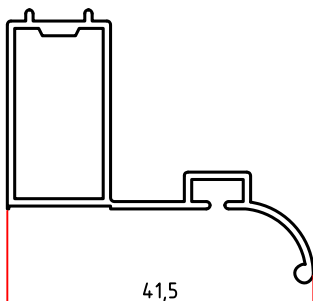
5087 0,373 Kg/m
