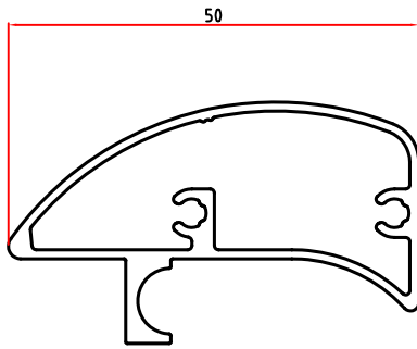
7190 0,588 Kg/m
