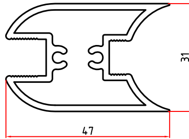
5320 0,980 Kg/m
