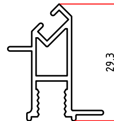
2706 0,310 Kg/m
