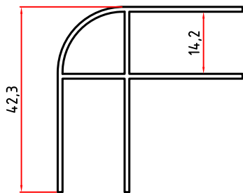
5071 0,496 Kg/m
