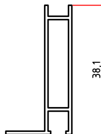
5106 0,289 Kg/m
