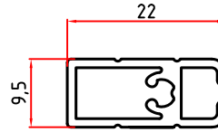
3184 0,239 Kg/m
