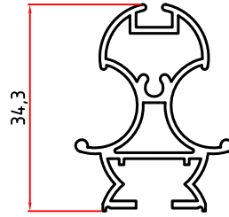
5064 0,442 Kg/m
