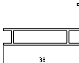
5076 0,299 Kg/m
