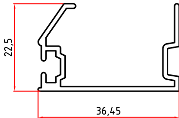
2703 0,347 Kg/m
