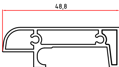
6163 0,527 Kg/m
