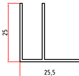
5081 0,209 Kg/m
