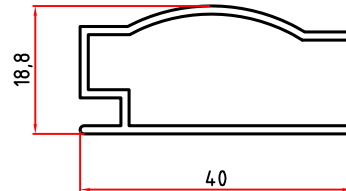
5663 0,342 Kg/m
