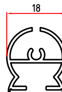
5070 0,228 Kg/m
