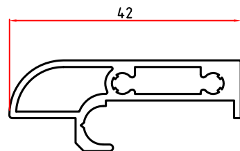
5889 0,476 Kg/m
