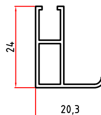
5074 0,214 Kg/m
