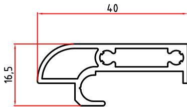
5664 0,441 Kg/m
