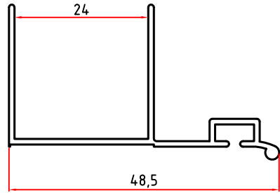
5271 0,320 Kg/m
