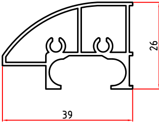
5031 0,532 Kg/m
