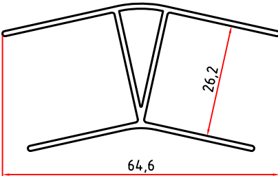
5033 0,586 Kg/m
