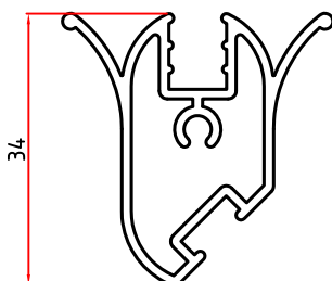
3092 0,522 Kg/m
