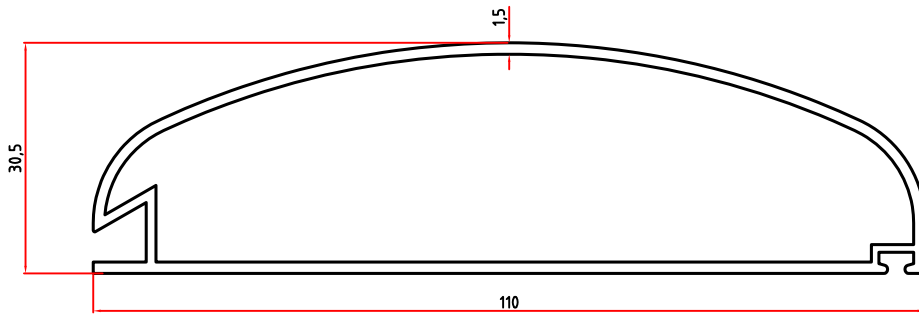
5216 1,105 Kg/m
