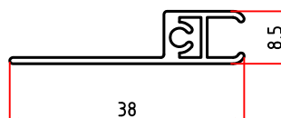
5078 0,213 Kg/m
