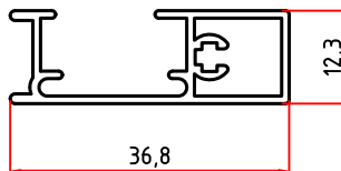
5072 0,313 Kg/m
