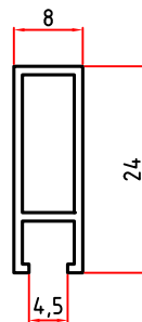
5080 0,175 Kg/m
