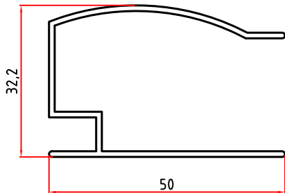
5886 0,469 Kg/m
