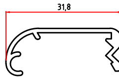
1738 0,226 Kg/m
