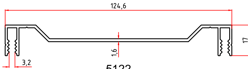
5122 0,842 Kg/m
