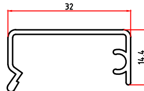
3295 0,236 Kg/m ( 3438 )
