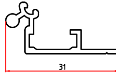
4225 0,219 Kg/m
