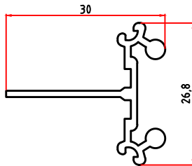
3438 0,298 Kg/m ( 3295 )
