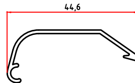
2302 0,230 Kg/m ( 2301- 4071-2841-4226-6147-5166 )
