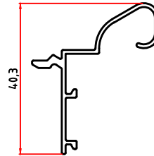
4935 0,279 Kg/m ( 4924-4925-4923-4926 )
