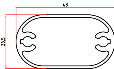
4156 0,571 Kg/m
