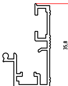
5235 0,345 Kg/m
