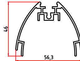
5131 0,796 Kg/m
