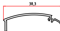
3405 0,153 Kg/m ( 3404 )
