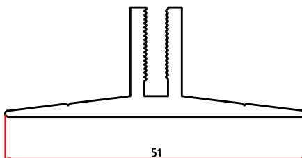
3673 0,567 Kg/m
