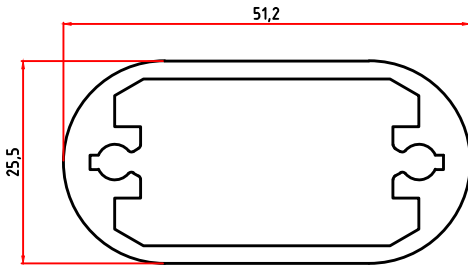
2303 1,119 Kg/m
