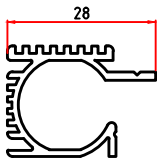
4730 0,368 Kg/m
