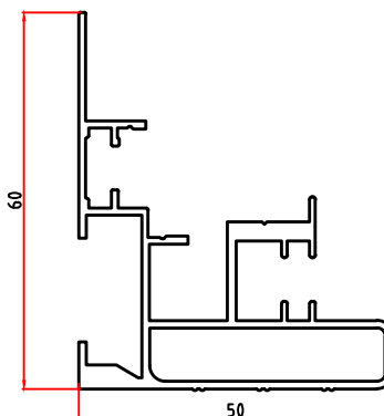
5356 0,922 Kg/m
