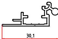
6051 0,210 Kg/m ( 6052 )
