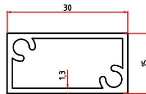
1562 0,378 Kg/m
