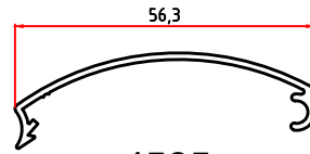
4585 0,283 Kg/m ( 4586 )
