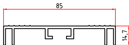
3666 0,834 Kg/m
