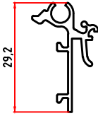
4926 0,244 Kg/m ( 4924-4925-4923-4935 )
