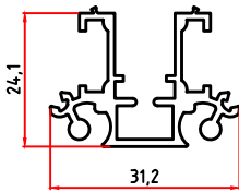
5102 0,550 Kg/m ( 5103 )
