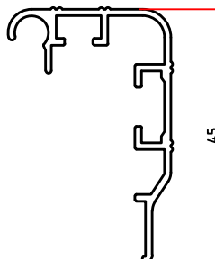
5234 0,388 Kg/m
