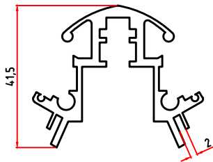
2890 1,075 Kg/m ( 2891 )
