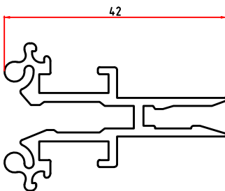
7026 0,646 Kg/m ( 7027 )
