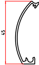
5870 0,250 Kg/m ( 5102 )
