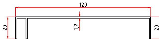
5115 0,574 Kg/m
