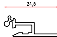
3667 0,145 Kg/m ( 2785 )
