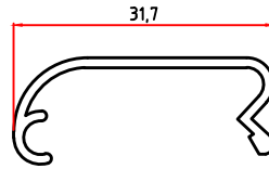
4147 0,199 Kg/m ( 1739-4329-2301-2841-4226-6147-4328 )
