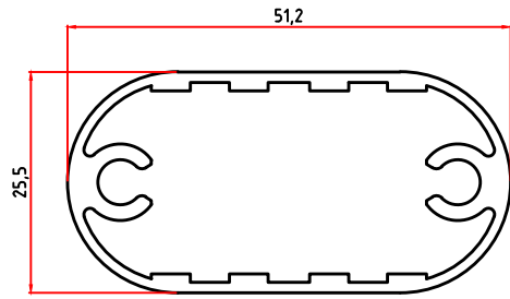
5233 0,748 Kg/m
