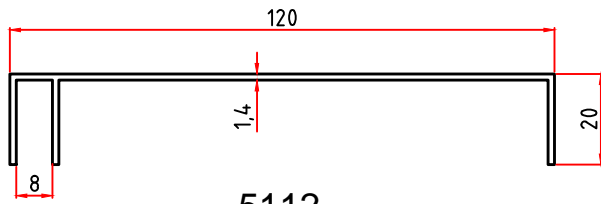
5112 0,667 Kg/m
