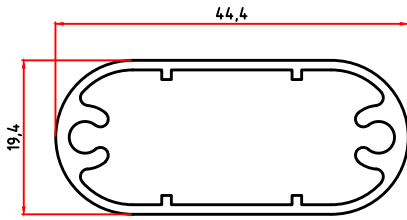
4177 0,522 Kg/m
