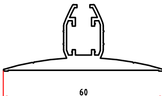
5264 0,769 Kg/m
