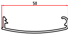
4894 0,272 Kg/m ( 4894 )
