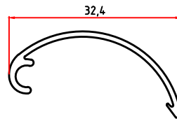
5240 0,156 Kg/m
