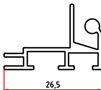
4927 0,250 Kg/m ( 4928 )
