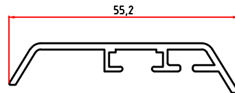
5754 0,371 Kg/m
