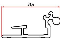
4328 0,253 Kg/m ( 1738-4147 )
