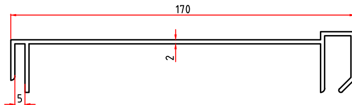
6444 1,533 Kg/m
