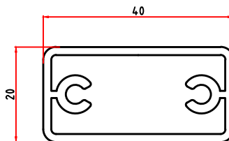
2304 0,719 Kg/m
