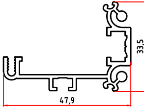
4586 0,606 Kg/m ( 4585 )
