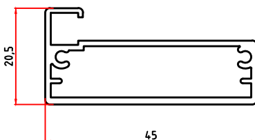
3286 0,519 Kg/m
