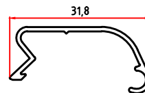
6052 0,168 Kg/m ( 6051 )
