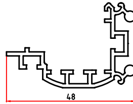
4895 0,645 Kg/m ( 4895 )
