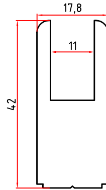
2201 1,461 Kg/m
