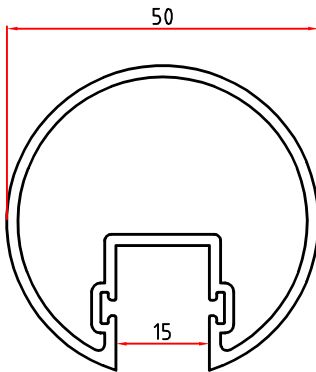
6413 1,016 Kg/m
