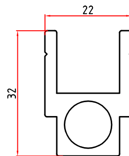
2193 0,780 Kg/m
