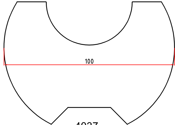
4037 14,142 Kg/m
