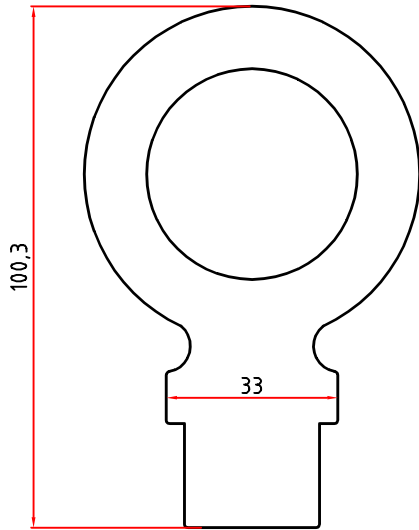
3471 8,525 Kg/m
