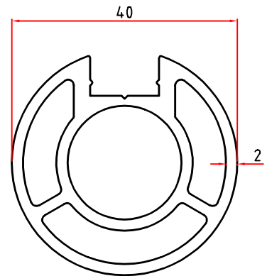
3874 1,206 Kg/m
