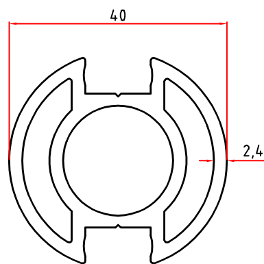
2504 1,315 Kg/m
