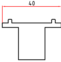
6535 1,503 Kg/m
