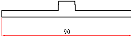
3447 1,366 Kg/m
