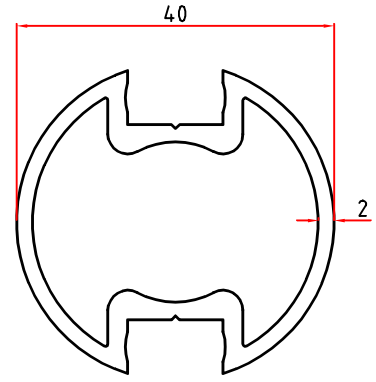
2105 0,931 Kg/m
