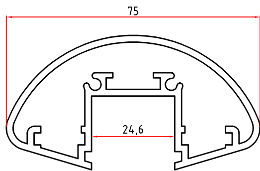
6423 1,469 Kg/m
