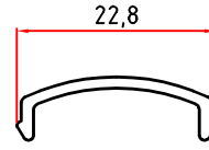
2195 0,114 Kg/m
