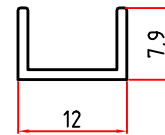
5683 0,080 Kg/m
