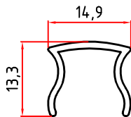
5542 0,124 Kg/m
