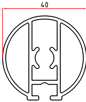
2958 0,989 Kg/m
