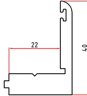
5501 1,093 Kg/m
