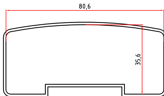
5685 0,870 Kg/m
