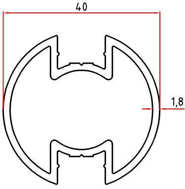
5266 0,808 Kg/m
