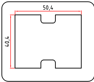
4064 6,623 Kg/m
