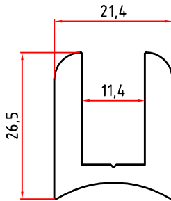
2733 0,810 Kg/m
