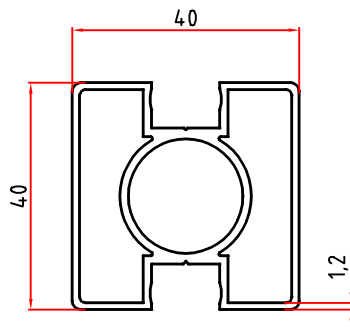
5682 0,953 Kg/m
