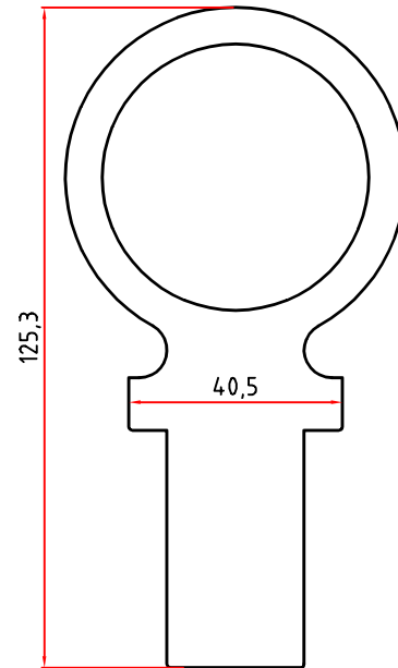
3942 8,613 Kg/m
