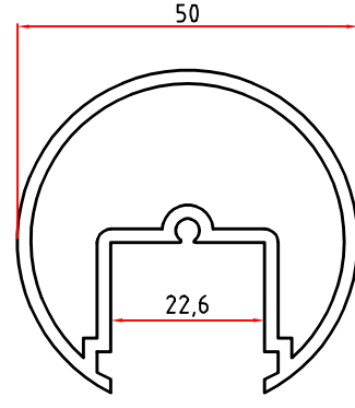
6425 1,121 Kg/m
