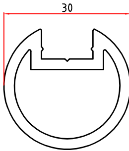
4525 0,700 Kg/m
