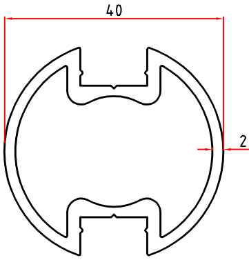
2839 0,914 Kg/m
