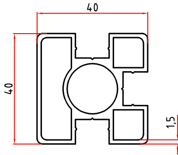
6504 1,151 Kg/m
