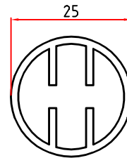
5730 0,450 Kg/m
