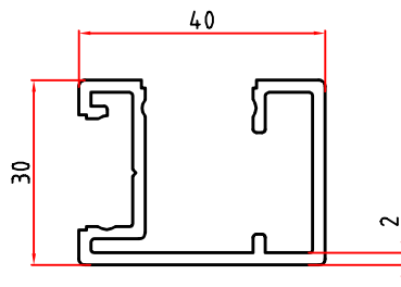
4227 0,773 Kg/m
