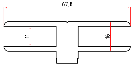
6657 1,532 Kg/m
