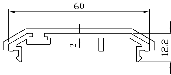
2352 0.507 kg/m
