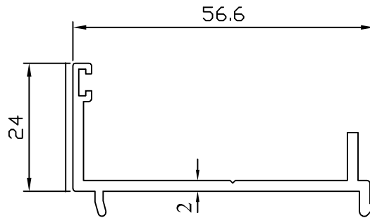
2353 0.542 kg/m
