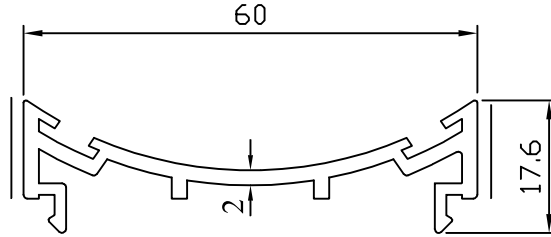
2351 0.618 kg/m
